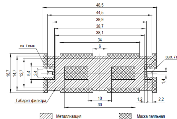
Рис.2 - Рекомендуемые размеры посадочного места для монтажа изделия пайкой на пасту паяльную на печатную плату FR4 IPC4101 толщиной 0,8 мм. Предусмотреть "земляные" металлизированные отверстия.
