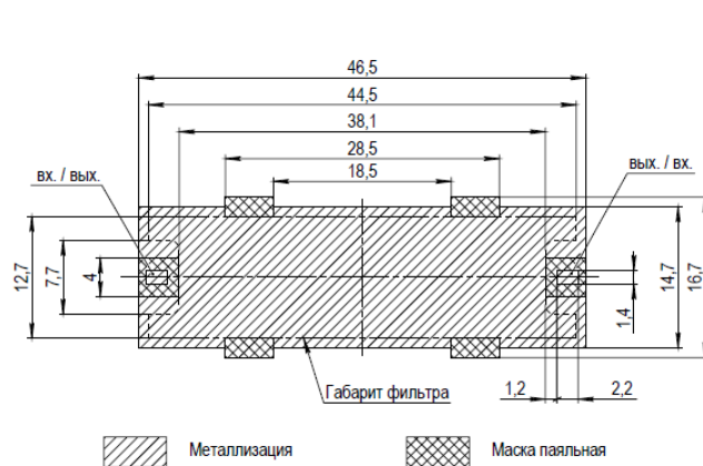
Рис.1 - Рекомендуемые размеры посадочного места для монтажа изделия пайкой по контуру на пасту паяльную на печатную плату FR4 IPC4101 толщиной 0,8 мм. Предусмотреть "земляные" металлизированные отверстия.
