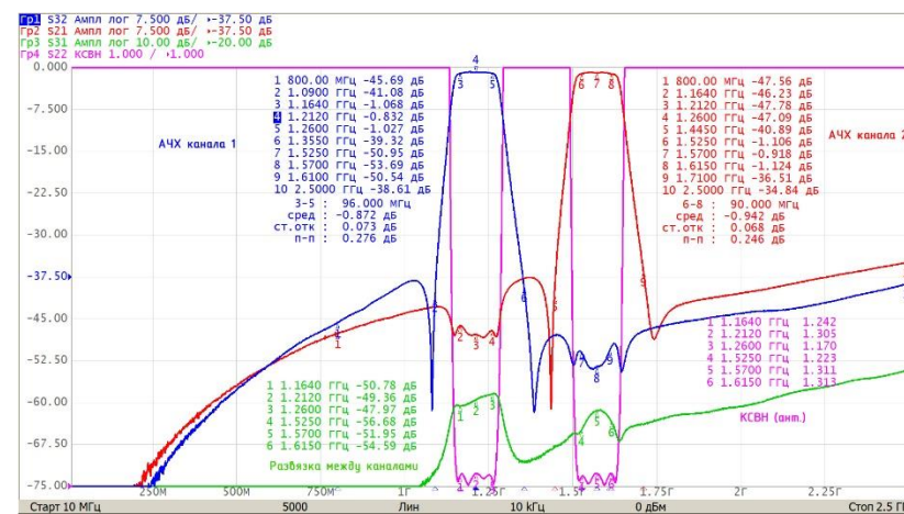
Характеристики каналов.
