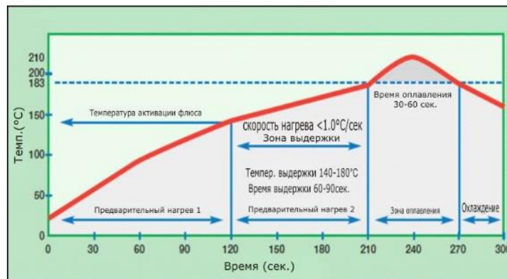
Рисунок 1. Термопрофиль оплавления пасты паяльной
